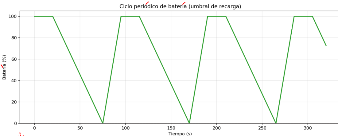
Fig. 5. Ciclo de batería periódico
